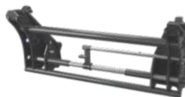
MX-werktuigadapter voor Euro-snelwisselframe
